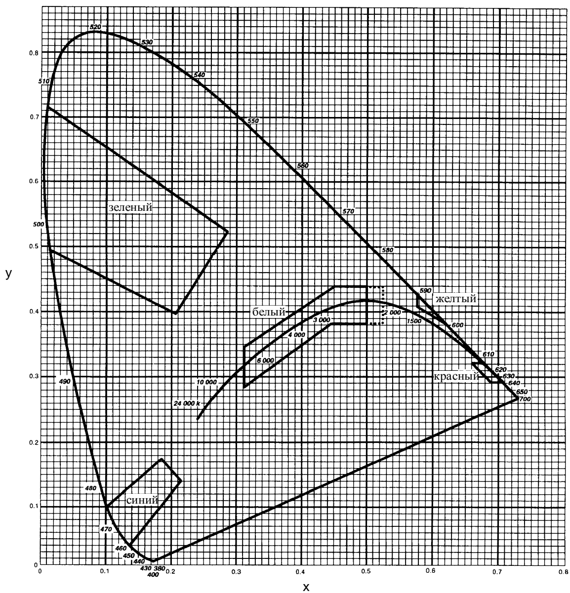
Рис.1 Диаграмма цветности МКС
